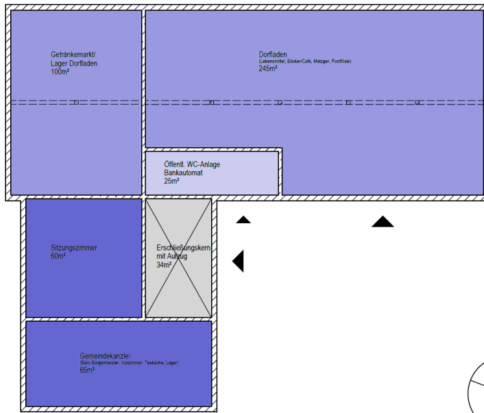
GRUNDRISS ERDGESCHOSS
